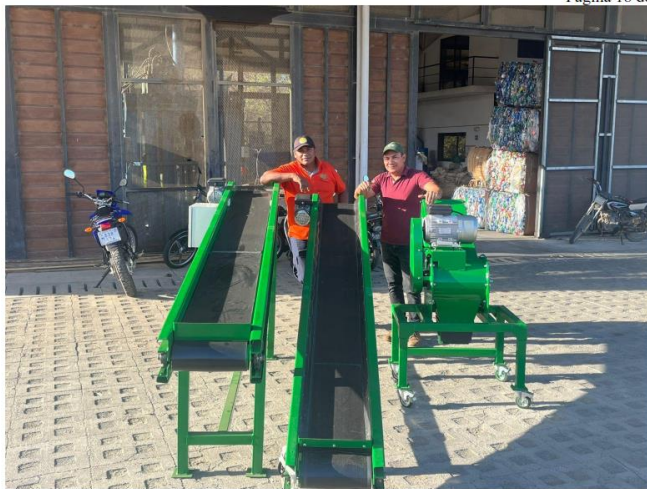
Figura 23. Trituradora de vidrio recibida con detalle de bandas transportadoras de material.
