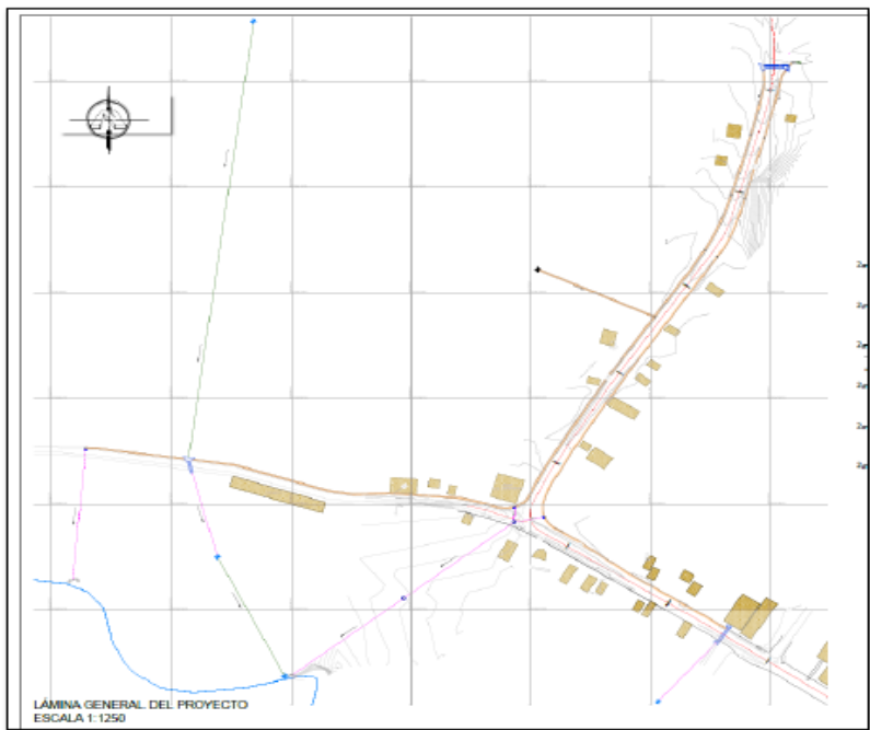
Imagen 1. Diseño de Canalización de aguas Pluviales de Río Grande, Lámina general del proyecto. Elaborado por: SETEIC S.A.
