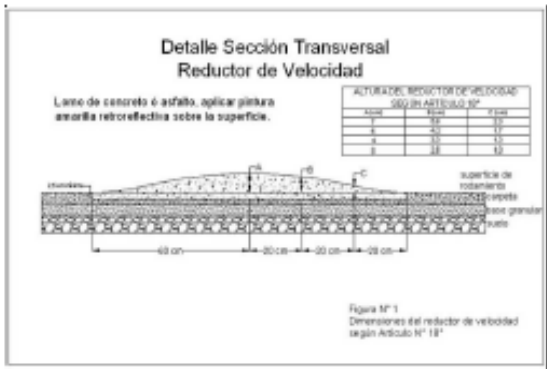
Figura 5. Detalle sección transversal del reductor de velocidad
