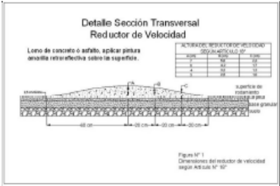
Figura 3. Detalle sección transversal del reductor de velocidad
