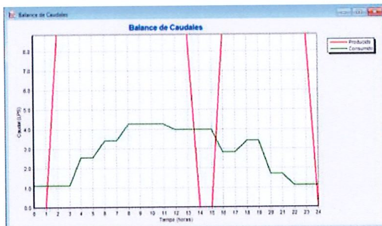
Figura 15. Balance de caudales, Sistema Aguas Frías
