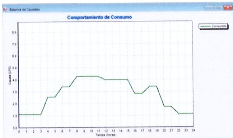
Figura 14. Hidrograma de consumo, Sistema Aguas Frías
