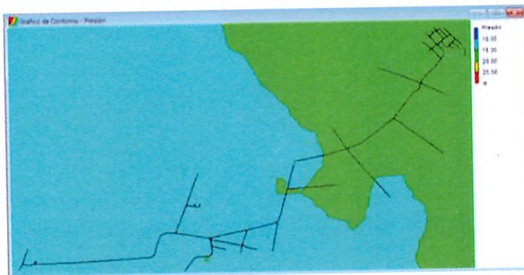
Figura 10. Mapa de presiones en condición de caudal coincidente Hidrante La Lidia al año 2048, Sistema Aguas Frías
