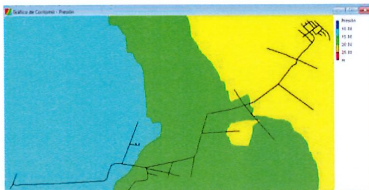
Figura 6. Mapa de presiones Caudal Máximo Diario 2022 incluyendo los tres nuevos proyectos, Sistema Aguas Frías
