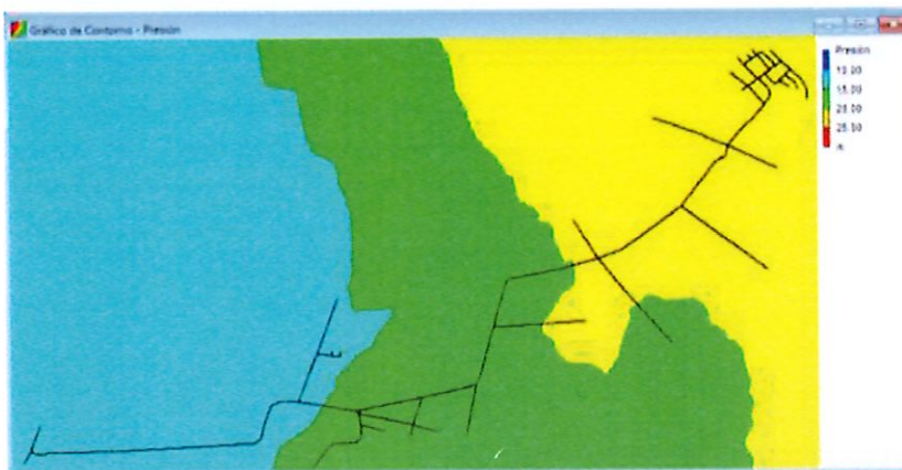
Figura 5. Mapa de presiones Caudal Máximo Diario 2023, Sistema Aguas Frías
