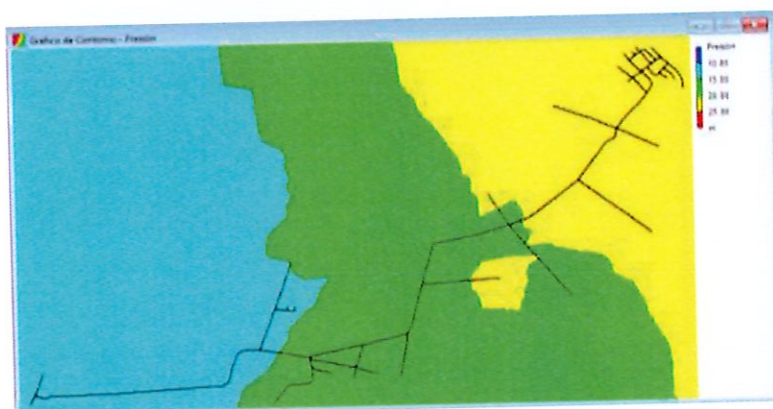
Figura 9. Mapa de presiones en condición demanda máxima diaria al año 2048, Sistema Aguas Frías
