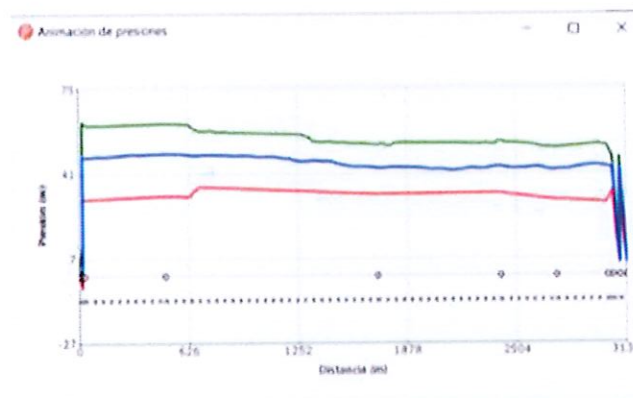
Figura 13. Grafica de Presiones línea impulsión Sistema Aguas Frías
