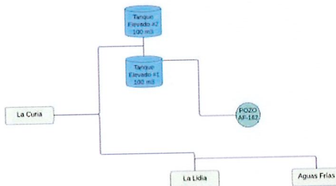
Figura 2. Esquema general del Acueducto de Aguas Frías
