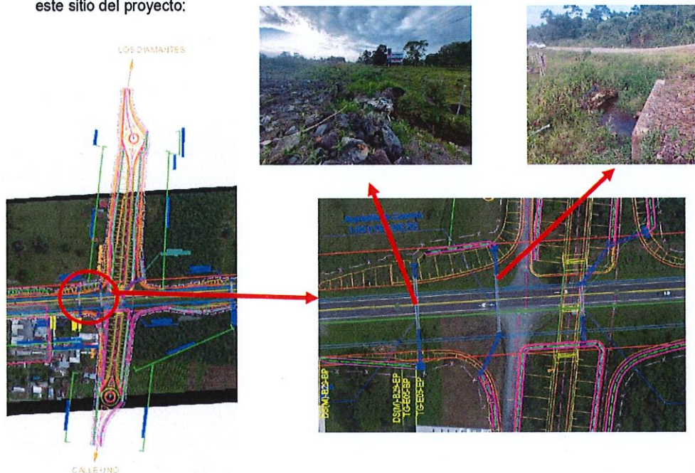
Diseño del PSV k64+600
