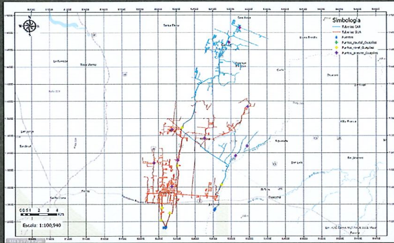
Mapa del actual sistema de acueducto.
