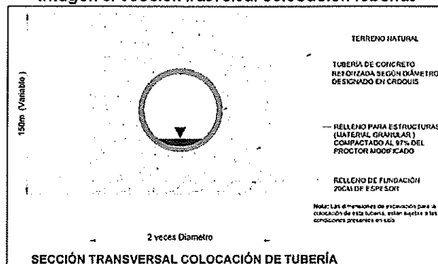
Imagen 4. Croquis sección transversal
