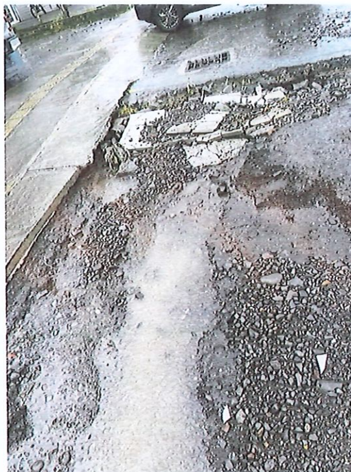
Foto 2. Lastre lavado por la escorrentía y carpeta asfáltica socavada aguas abajo de la alcantarilla.
