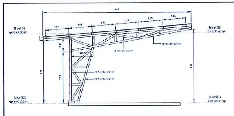
Figura 11.- Diseño estructural de la cubierta de techo de los parques
