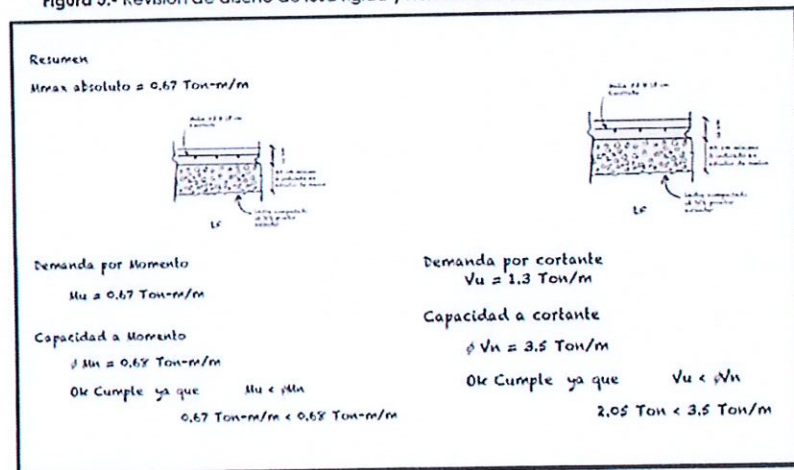
Figura 5.- Revisión de diseño de losa rígida y nervadura / Memoria de cálculo estructural
