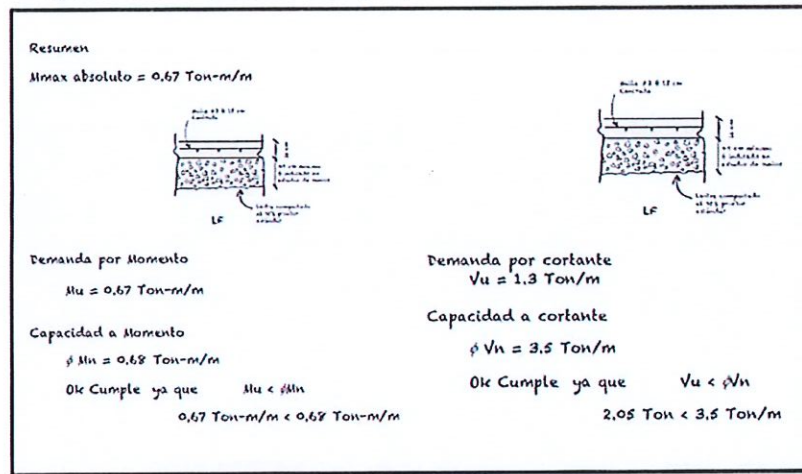
Figura 5.- Revisión de diseño de losa rígida y nervadura / Memoria de cálculo estructural
