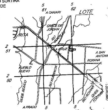
UBICACION GEOGRAFICA HOJA GUAPILES 3446-IV ESCALA 1:50000
