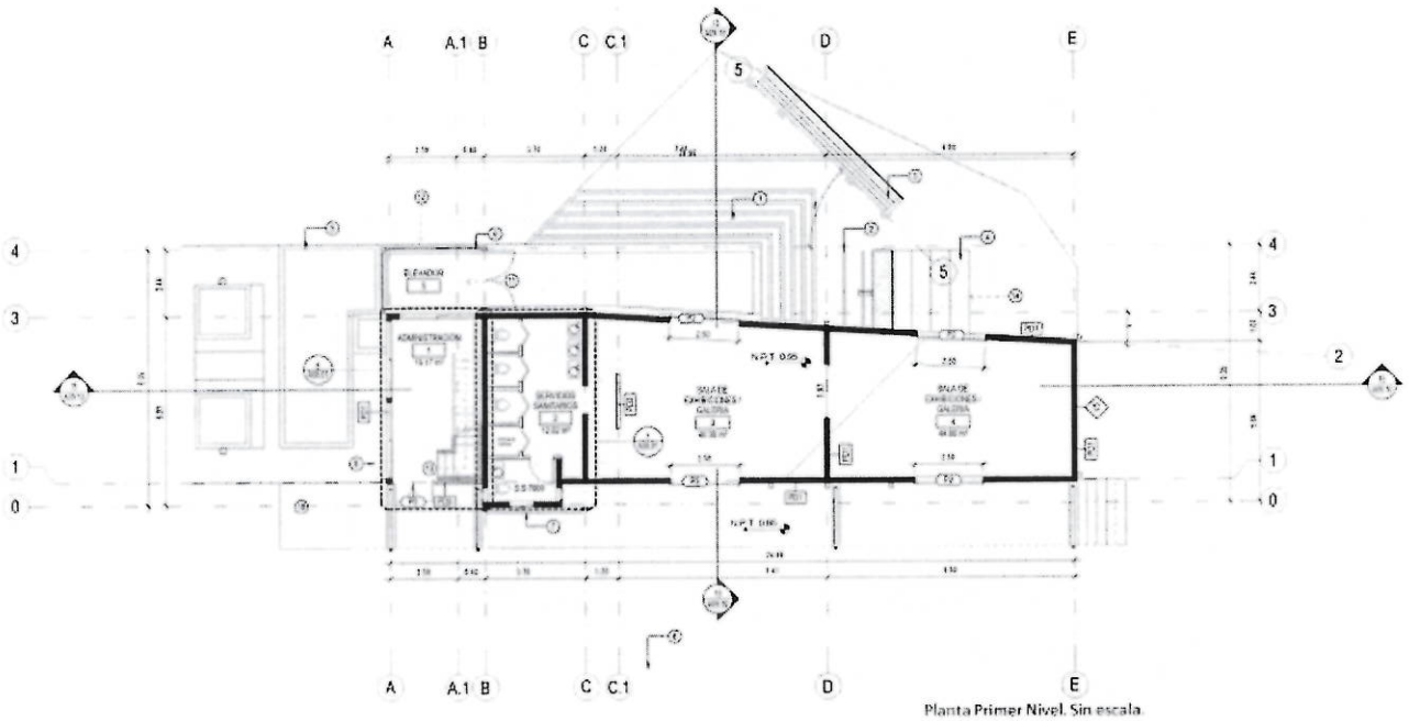
Planta Primer Nivel. Sin escala.
