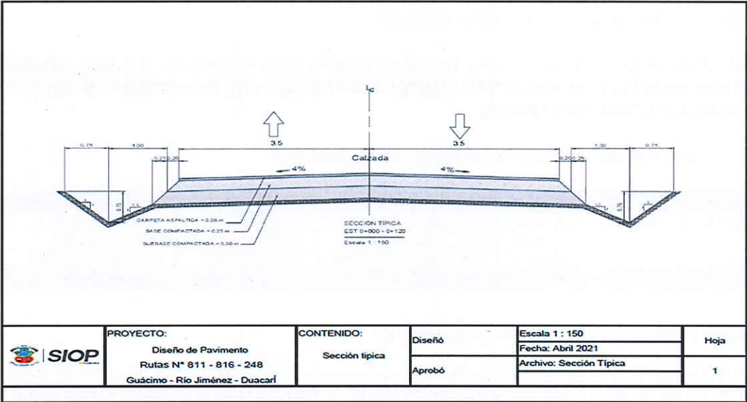
Cuadro 1. Diseño de la estructura de pavimento, RN 811-816-248
