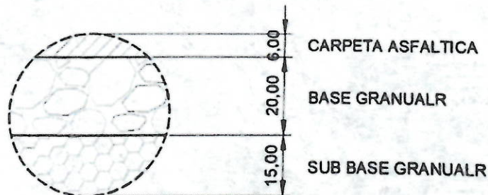
Figura 2. Detalle ampliado de la estructura de pavimento diseñada.
